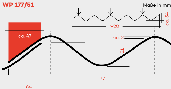
Querschnitt der PLEXIGLAS® Resist WP 177/51 (Maße in mm)
